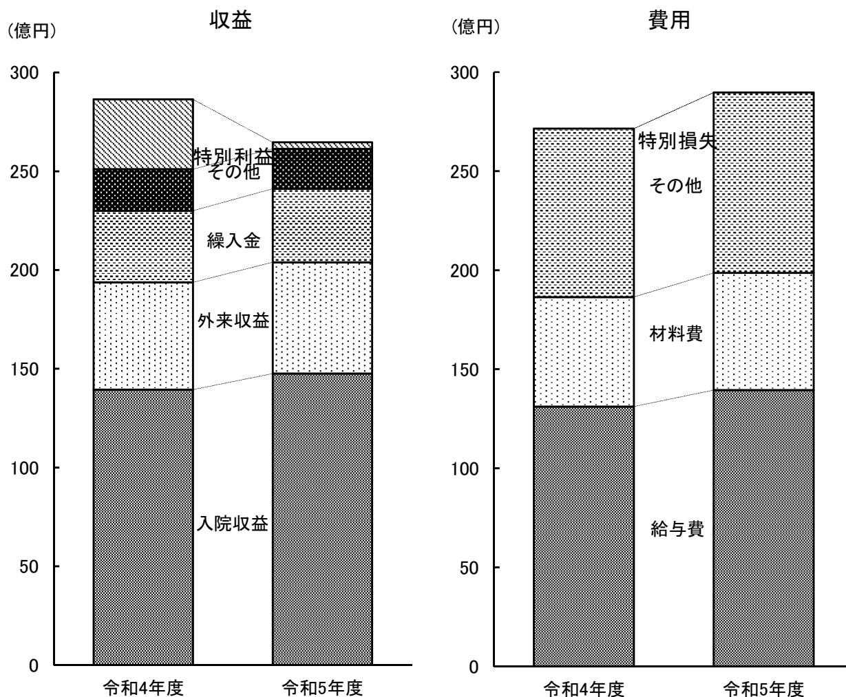
図6-1 収益費用
